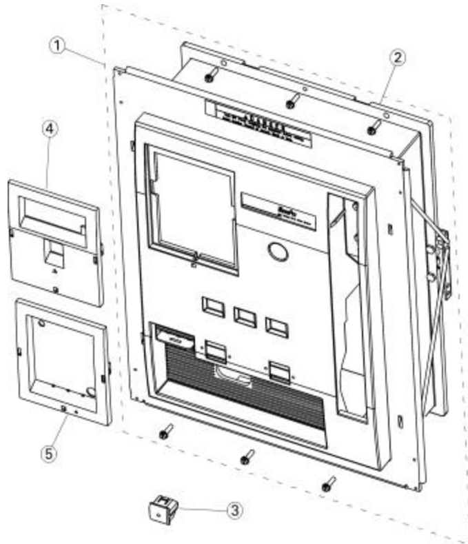
Figure 27. Escutcheon.
