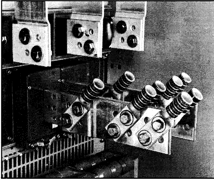
Figure 4-3 Lug Landings
