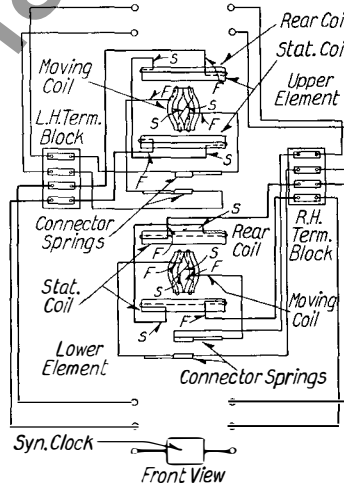
FIG. 15*—TYPE GY-40 POLYPHASE WATTMETER
