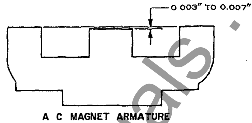
Fig. 30. Ac armature
