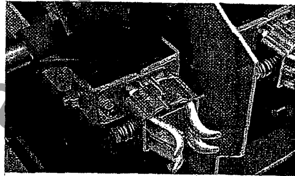
Fig. 37. Power-stab fingers
