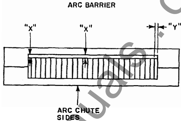
Fig. 22. Arc-chute dimensions
