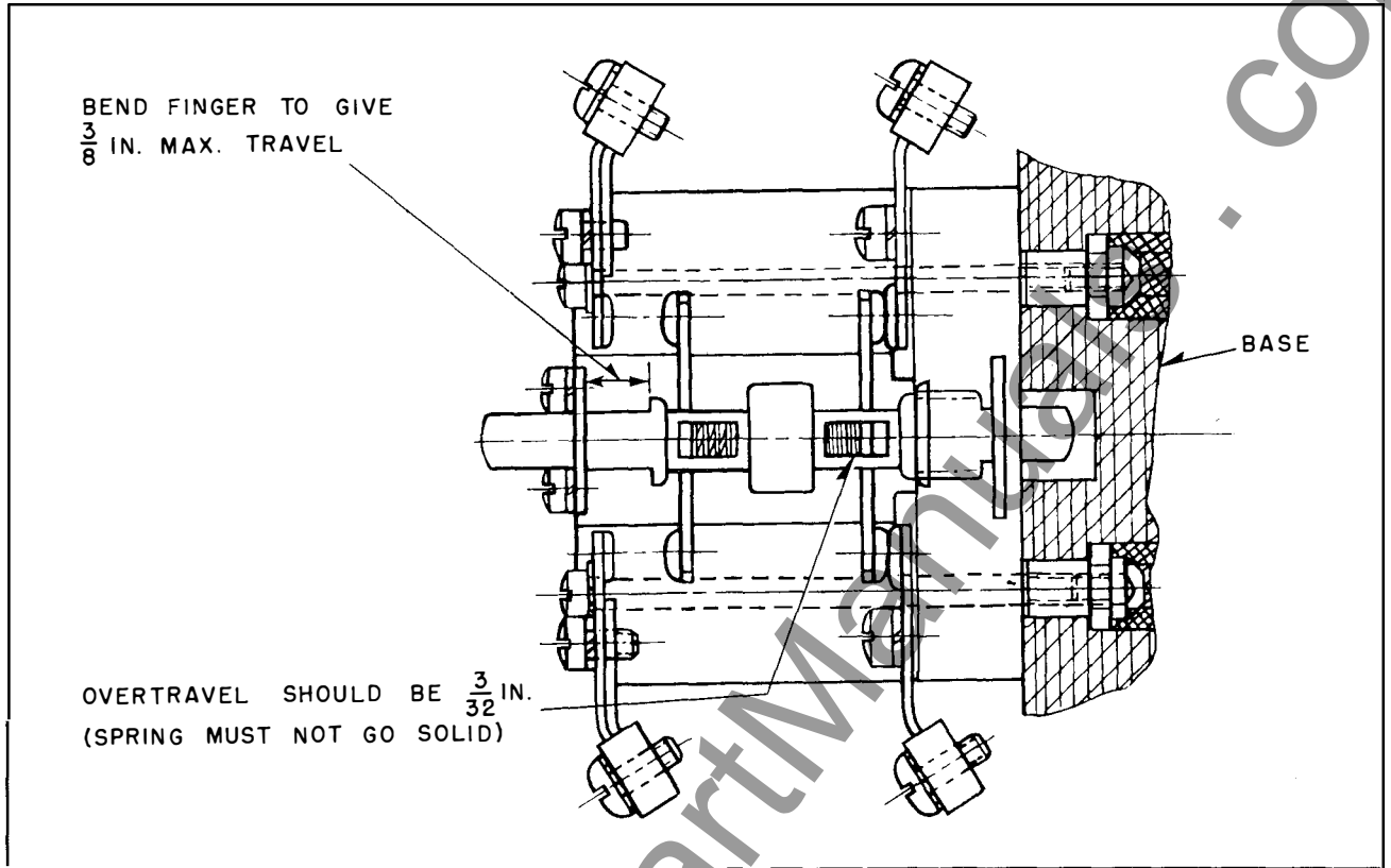
FIG. 12. L61 Electrical Interlock
