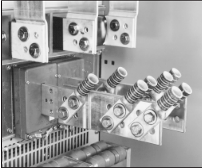
Figure 4-3 Lug Landings
