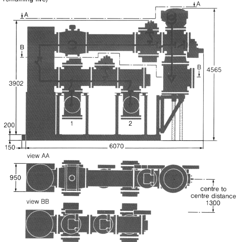
«Double busbar» bay, without «common point» compartment
