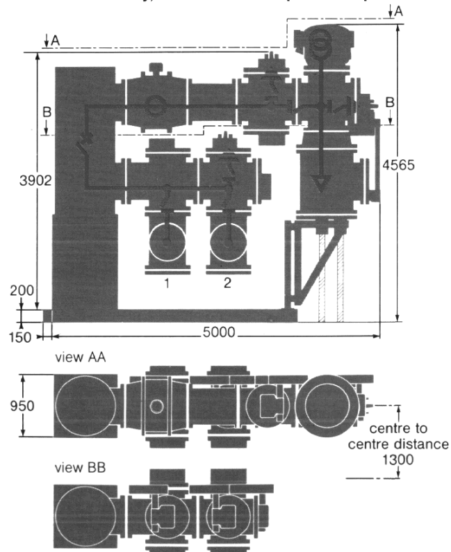
«Double busbar» bay, without «common point» compartment
