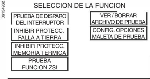
Figura 59: Pantalla "Selección de la función"
