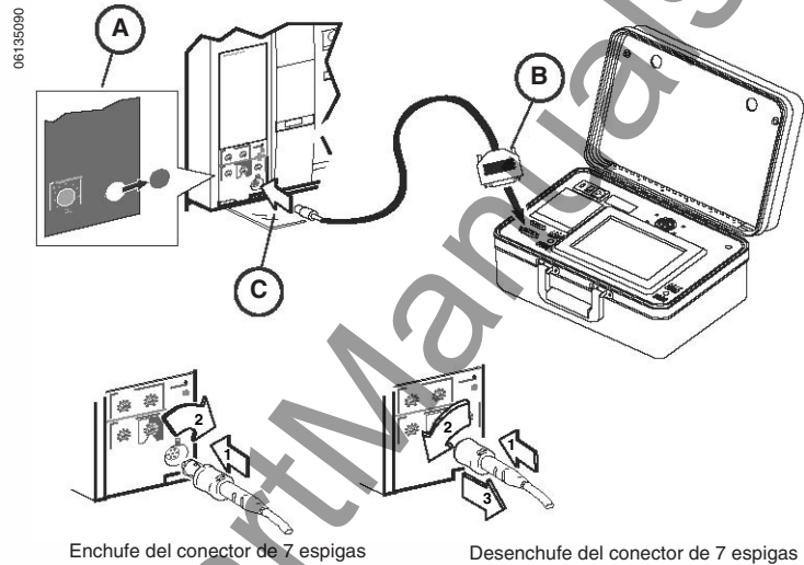
Figura 3: Conexión a las unidades de disparo Micrologic® y ET
