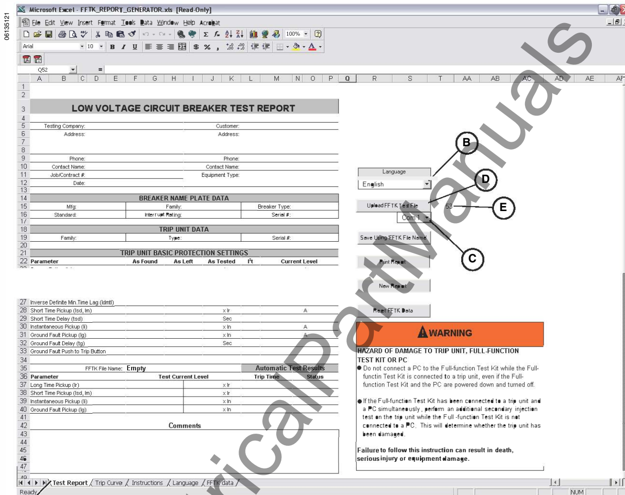
FIG. 4 : Test Report Tab / Ceja Informe de prueba / Onglet Rapport d'essais
