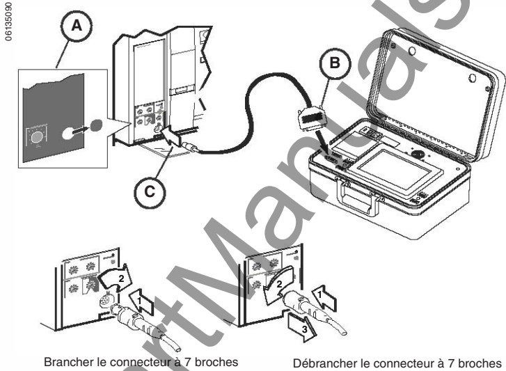
Figure 3 : Raccordement aux déclencheurs Micrologic et ET
