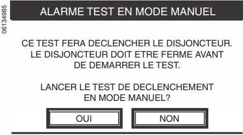
Figure 36 : Écran « Test en mode manuel »
