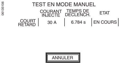
Figure 36 : Écran « Test en mode manuel »
