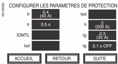
Figure 15 : Écran « Configurer les paramètres de protection »
