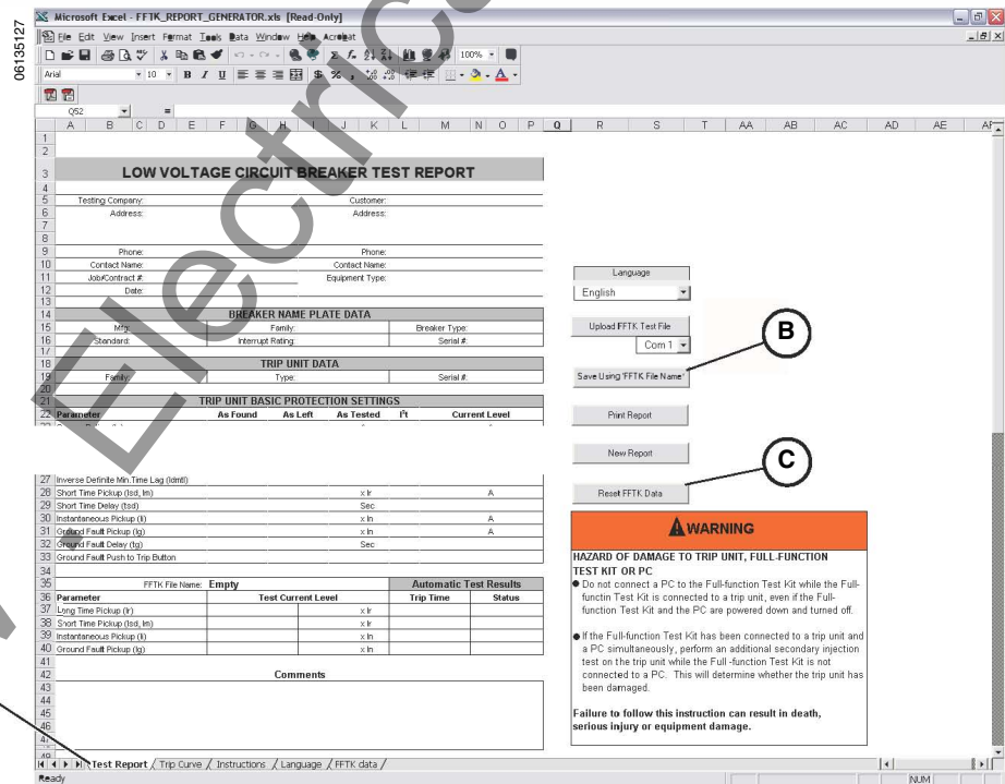
FIG. 8 : Saving a Test Report / Almacenamiento de un informe de prueba / Sauvegarde d'un rapport d'essai
