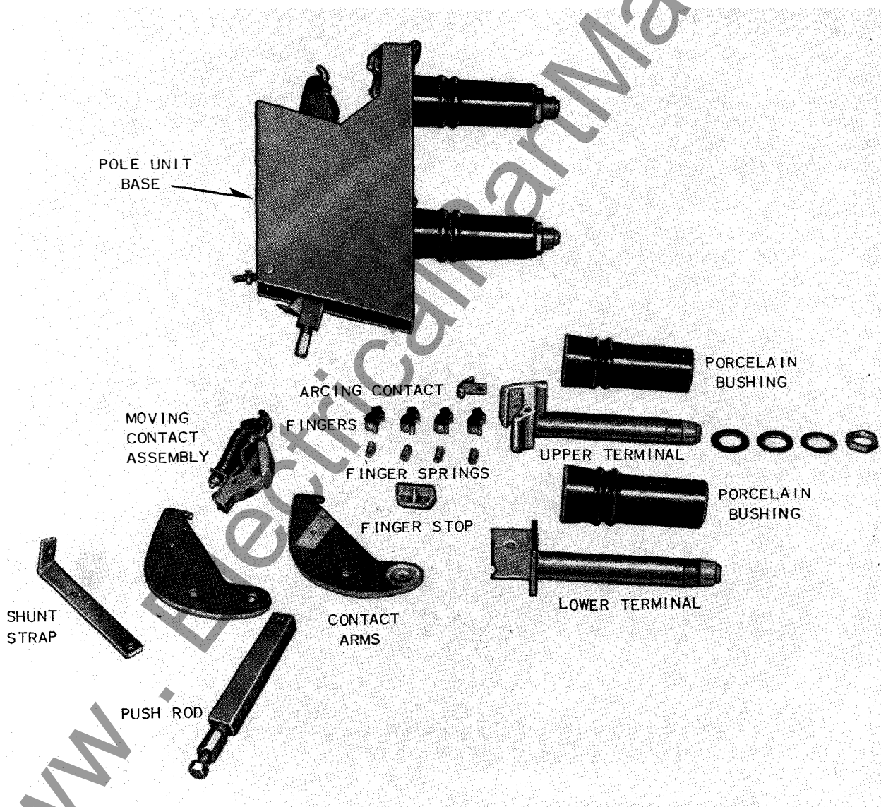
FIG. 8. Pole Unit Assembly
