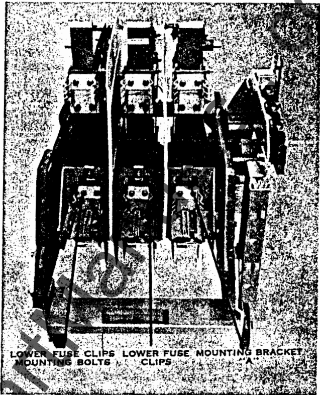
Fig. 25. IC2814E250 contactor
