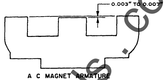
Fig. 30. Ac armature
