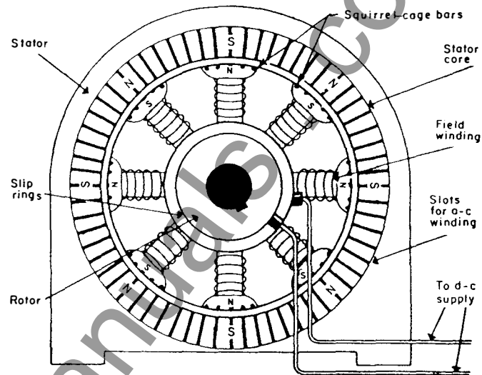
Fig. 1. Salient-pole synchronous motor
