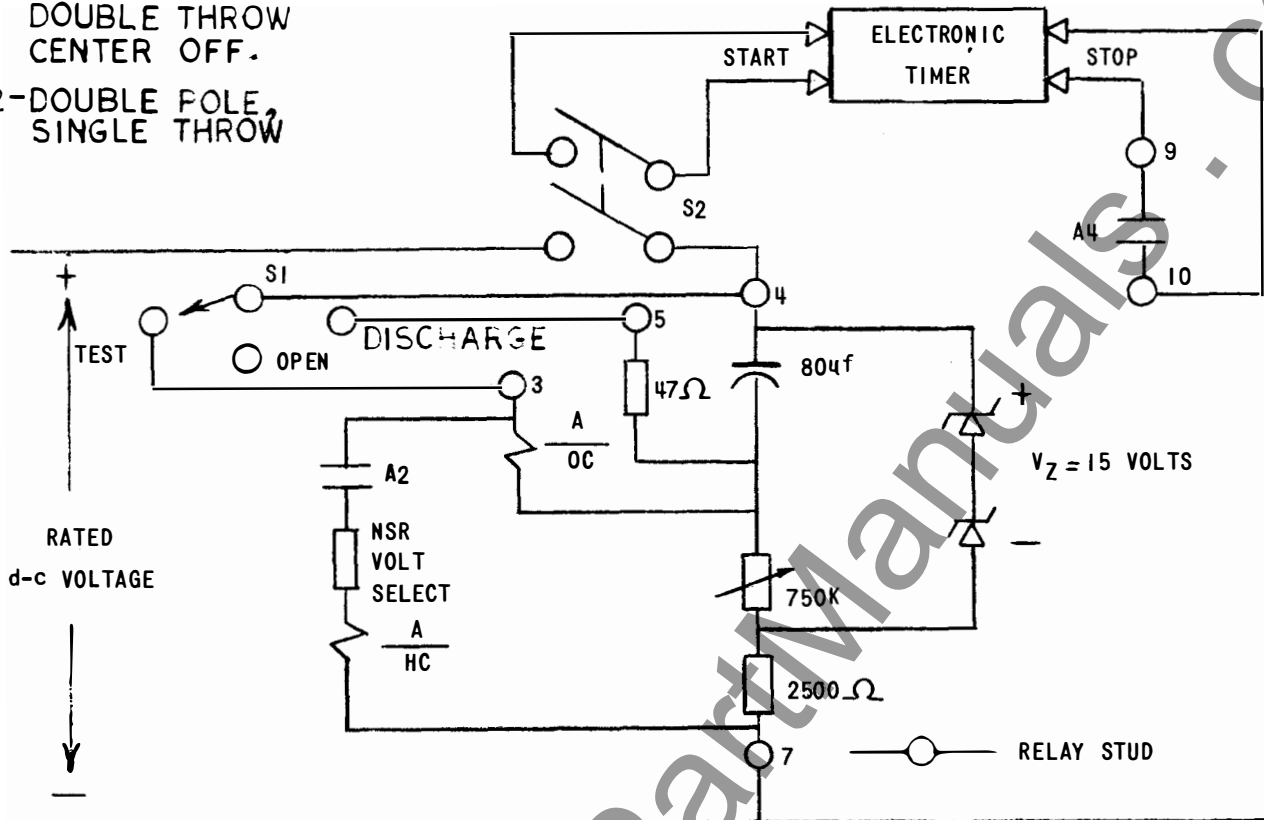
a. SCHEMATIC
