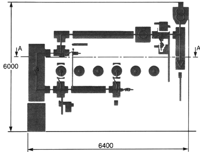
«Double busbar» bay - (busbar with one enclosure per phase)
