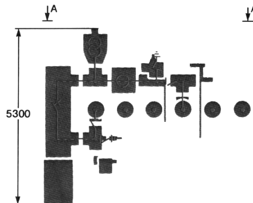
«Busbar coupling» bay
