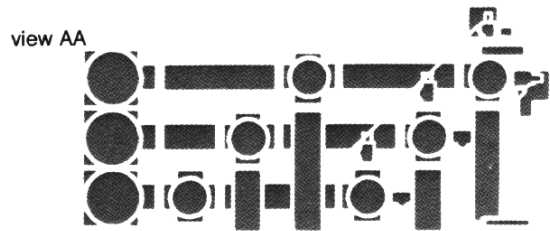
«Breaker and a half» bay
